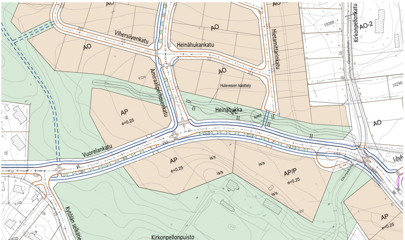
Kuva 14. Ote alueelle laaditusta katujen yleissuunnitelmasta Vuorelankadun osalta
