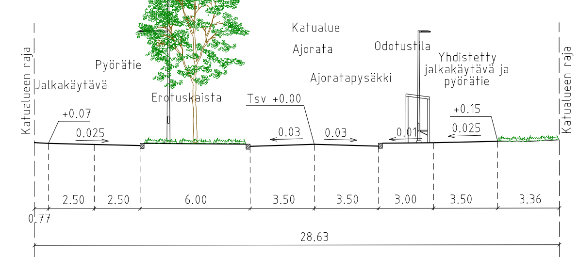
POIKKILEIKKAUS B - B 1:200
