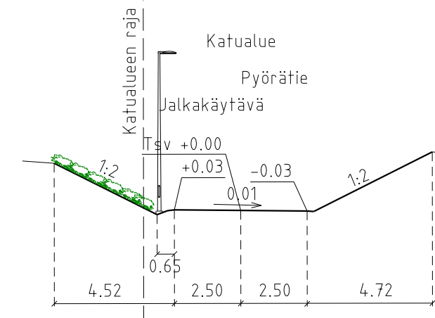
POIKKILEIKKAUS A - A 1:200
