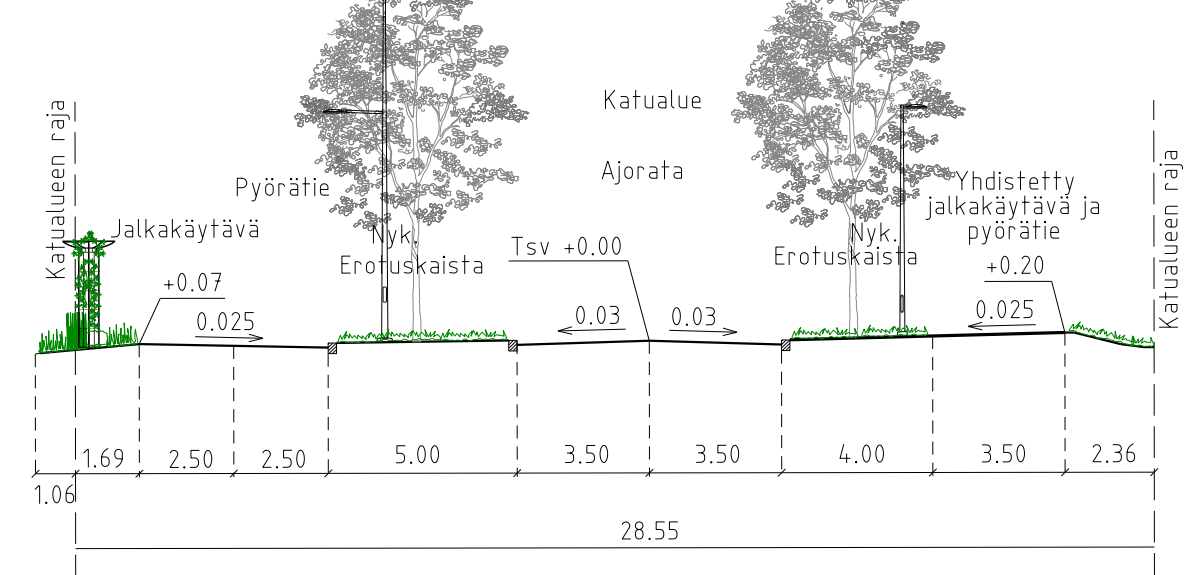
POIKKILEIKKAUS C - C 1:200
