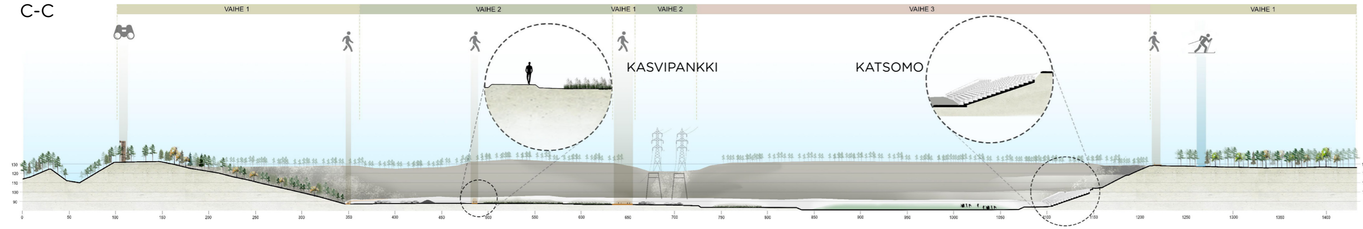
Poikkileikkaus C-C sorakuopan suuntaisesti kohti pohjoista.
