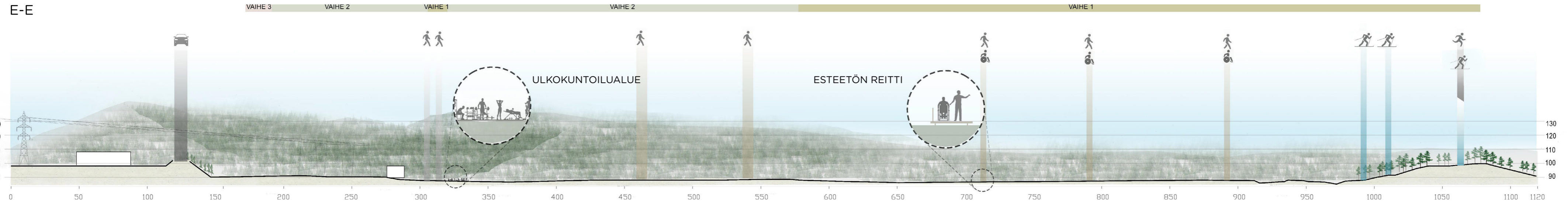
Poikkileikkaus E-E sorakuopan suuntaisesti kohti lounasta.
