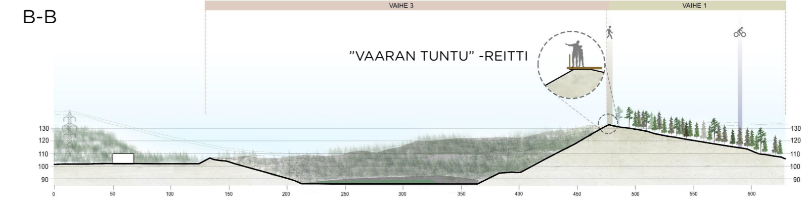
Poikkileikkaus B-B sorakuopan keskiosan poikki kohti länttä.
