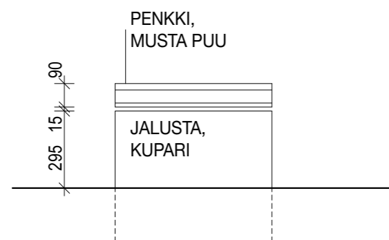
KALUSTE SIVULTA
