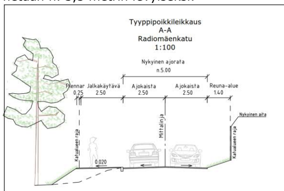
Kuva 10. Radiomäenkadun poikkileikkaus
