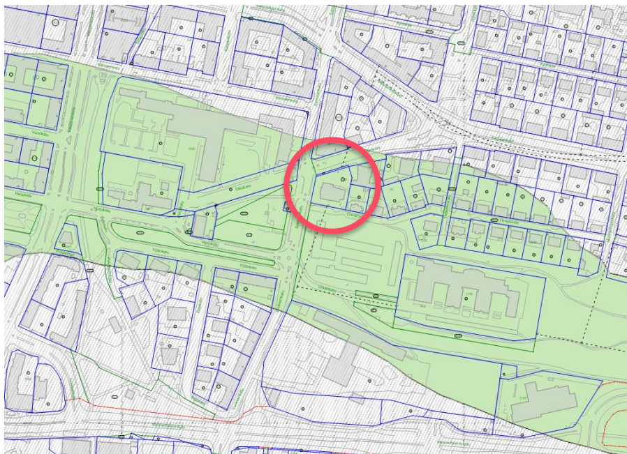
Maaperäkartta (GTK_WMS). Vihreä vyöhyke, jolla kaava-alue sijaitsee, on hiekkaa (Hk).
