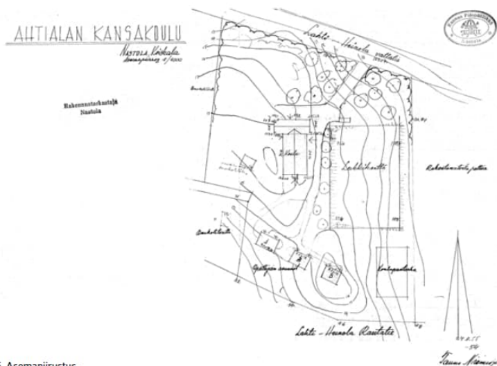
Kuva 5. Asemapiirustus.
